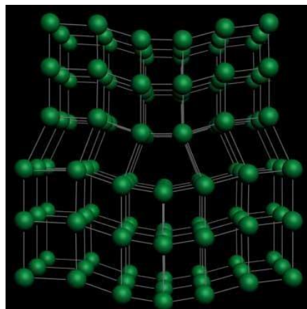
Fig 5. Edge dislocations
